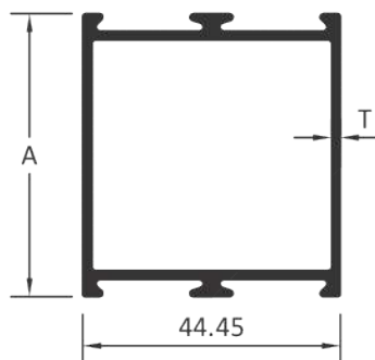
DOOR MIDDLE
