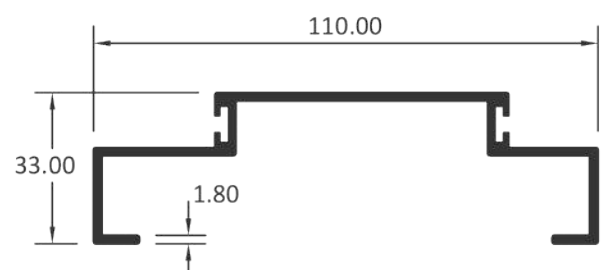
ART3007991 0.983 Kg/m
