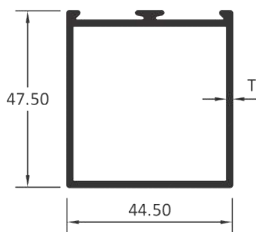
DOOR TOP
